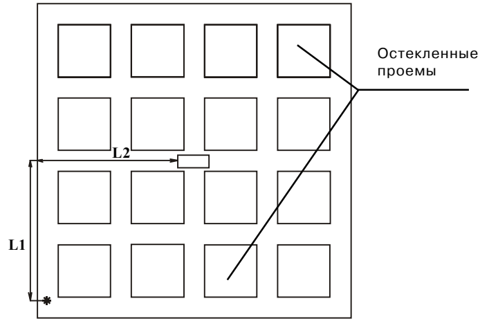
Рис.6 Защита переплета оконной рамы
